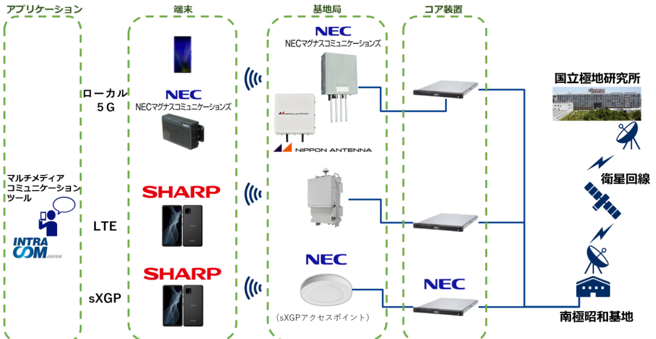
南極 昭和基地における実証実験系統図
